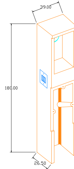
ISOMETRICO
