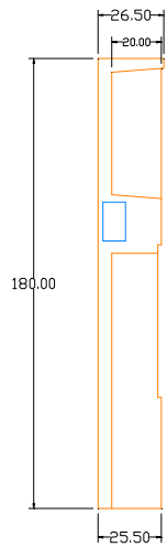
VISTA LATERAL
