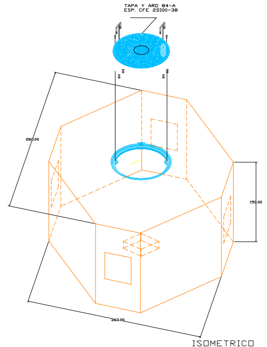
ISOMETRICO
