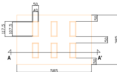
VISTA SUPERIOR
