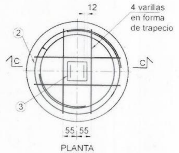
ANCLA CÓNICA C3
